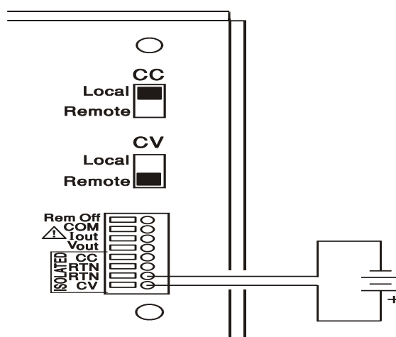
Commande de Courant Constant
