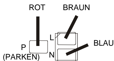
230V BETRIEB (VON OBEN GESEHEN)
